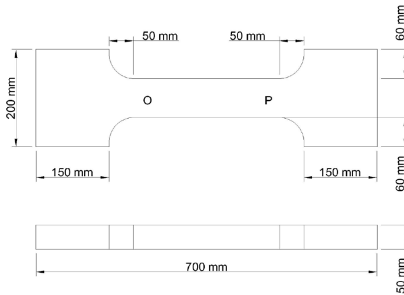
Fig. 6. Schéma des éprouvettes pour l'essai de traction directe
