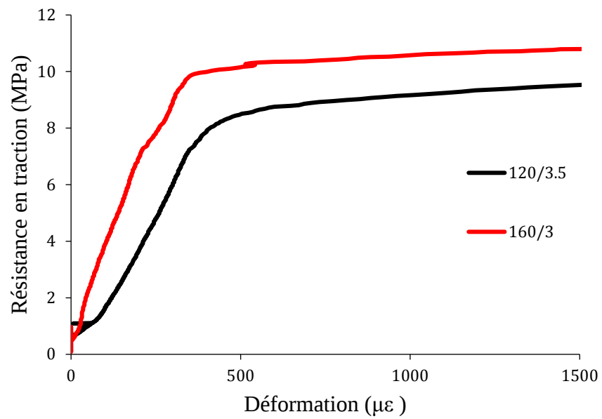
Fig. 8 Les courbes typiques de 2 mélanges caractérisés enregistrés de BFUP (résultats individuels)
