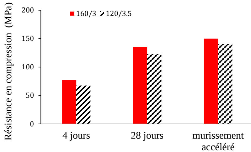
Fig. 4. Résistance en compression
