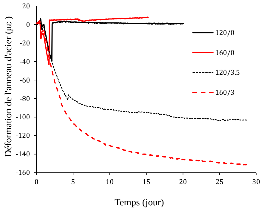
Fig. 11 Retrait restreint (sensibilité à la fissuration)
