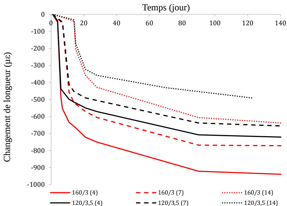
Fig. 10 Changement de longueur des éprouvettes soumise au séchage
