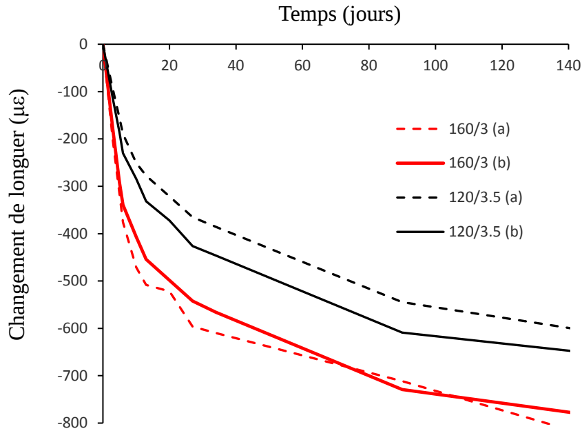
Fig. 9 Changement de longueur des éprouvettes scellées (retrait endogène)
