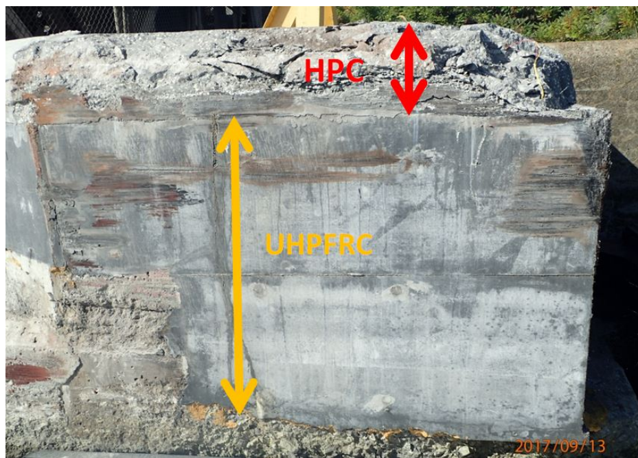
Fig. 14 Aspect du coin de mur réparé après une année en service
