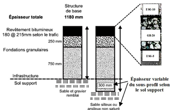
Figure 3 – Structure de chaussée type avec sous-profil en fonction du sol support
