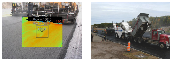
Figure 4 – A) Détection de ségrégation thermique par infrarouge B) Asphaltage avec utilisation d'un VTM
