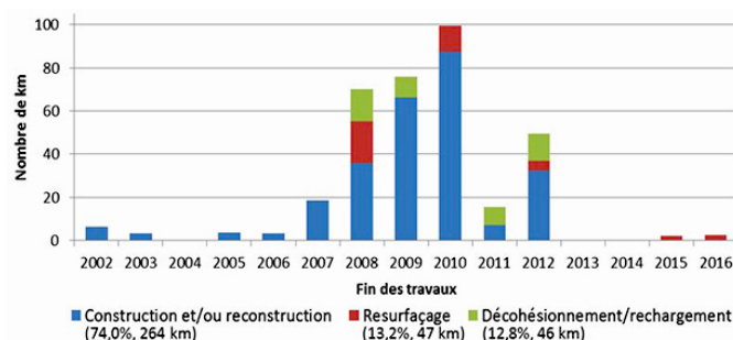
Figure 2 – Interventions sur la route 175 de 2002 à 2016
