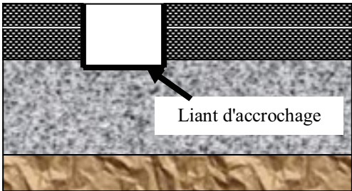
Figure 3 : Sciage, nettoyage et application d'un liant d'accrochage
