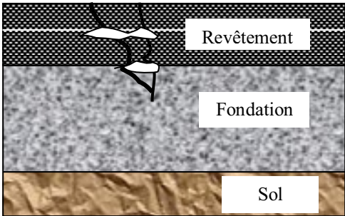
Figure 1 : Infiltration d'eau
