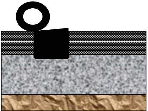
Figure 4 : Pose et compactage de l'enrobé
